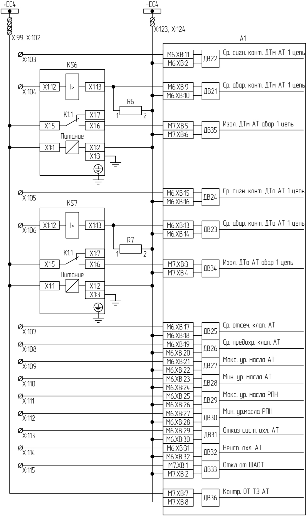
Цепи оперативного тока ТЗ АТ А1
